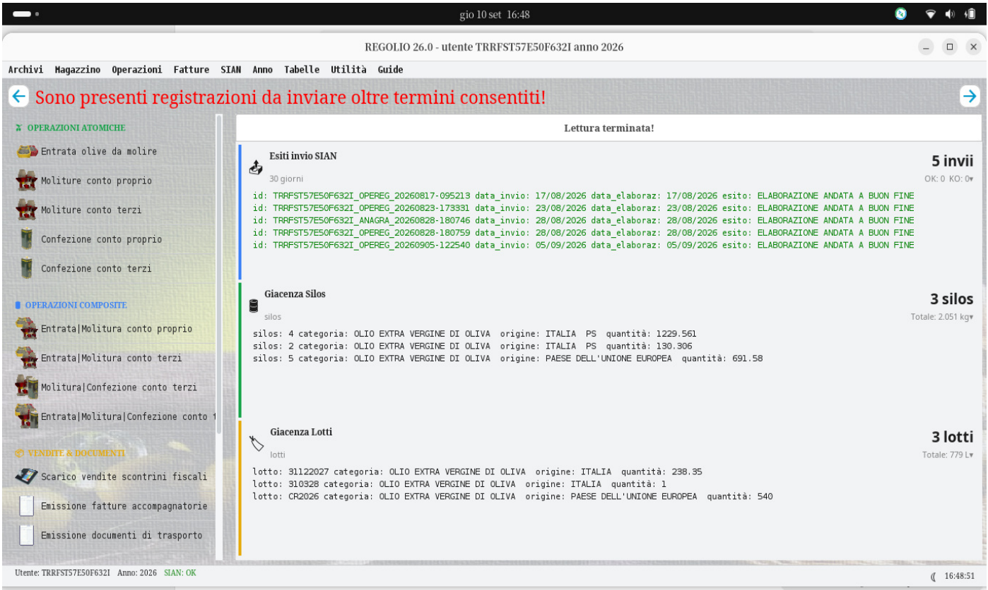
La schermata principale: scorciatoie alle operazioni, esiti SIAN e giacenze in tempo reale.
